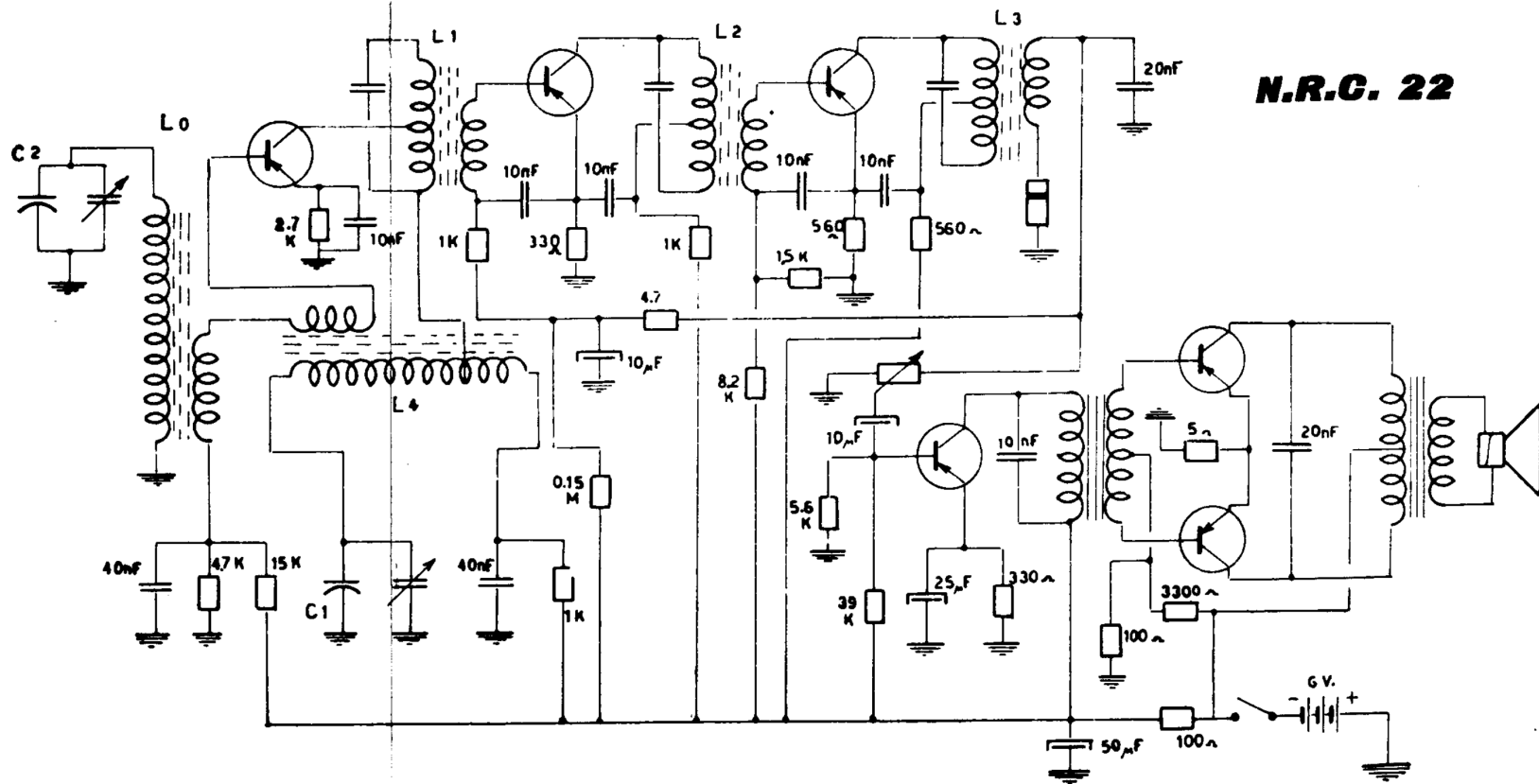
PRANDONI - Mod. NRC 22. Apparecchio portatile a transistor, con pannello a circuiti stampati. Antenna magnetica incorporata. Gamma onde medie. Media frequenza a 468 kc/s. Resa d'uscita 200 milliwatt.
